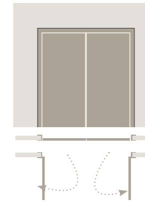
porta a battente hinged door porte à battant puerta batiente Flügeltür распашная дверь L 600/650/700/750/800/900 H 2000/2100
